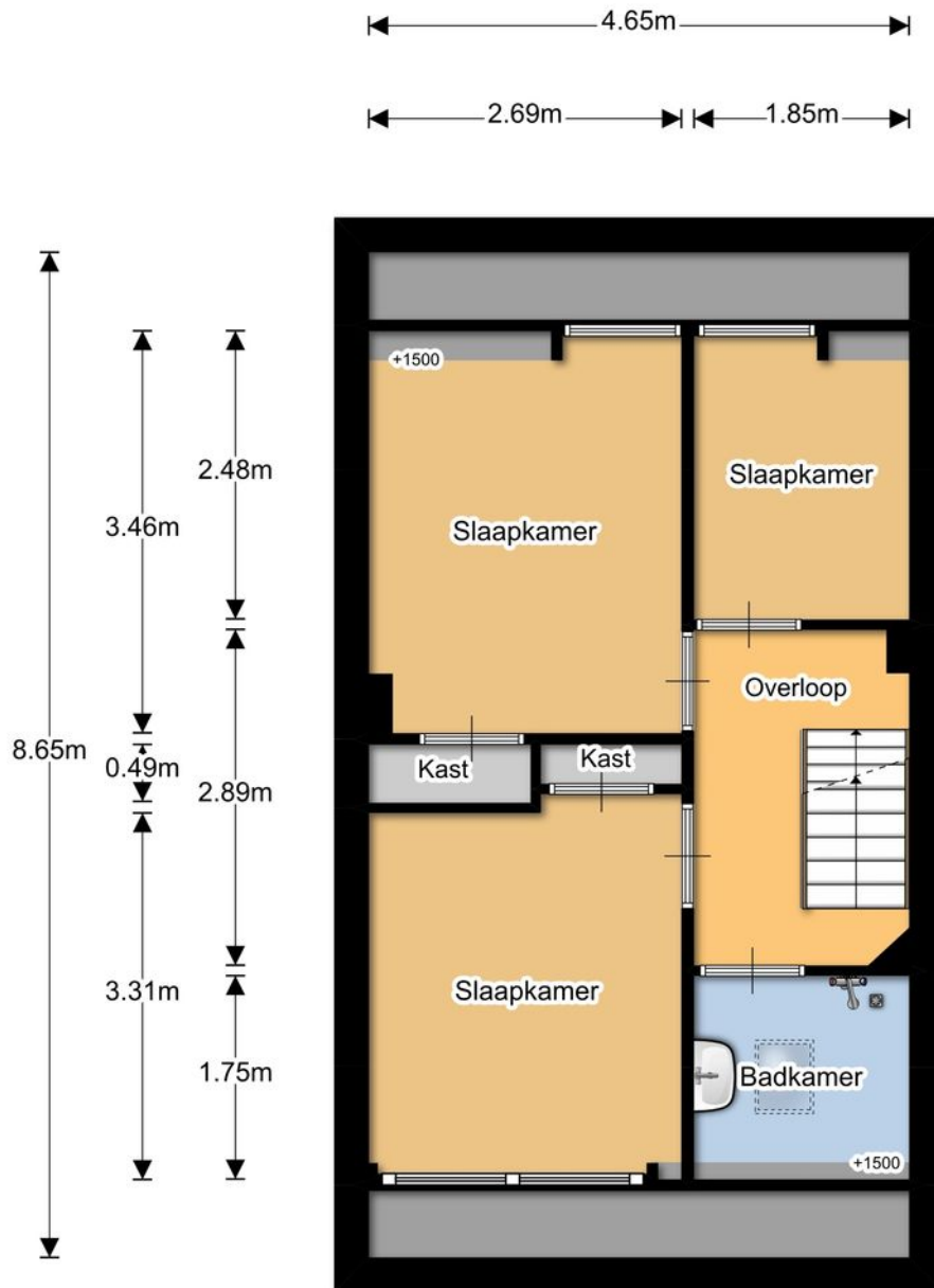
1e verdieping
